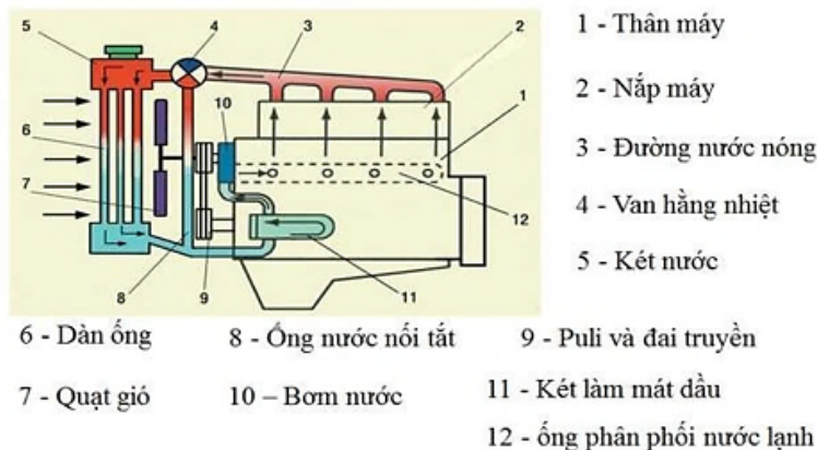
Hệ thống làm mát bằng nước loại tuần hoàn cưỡng bức Nguyên lý hoạt động dựa trên sơ đồ hệ thống làm mát bằng nước
